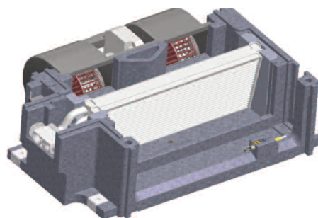
Модульна концепція випаровувача з плоскими тубами / Modular concept with flat-tube evaporator
