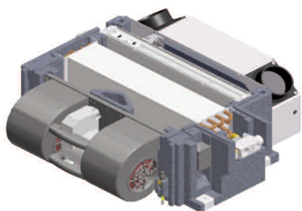
Модульна концепція з клімат-контролем / Modular concept with fully automatic air-heating
