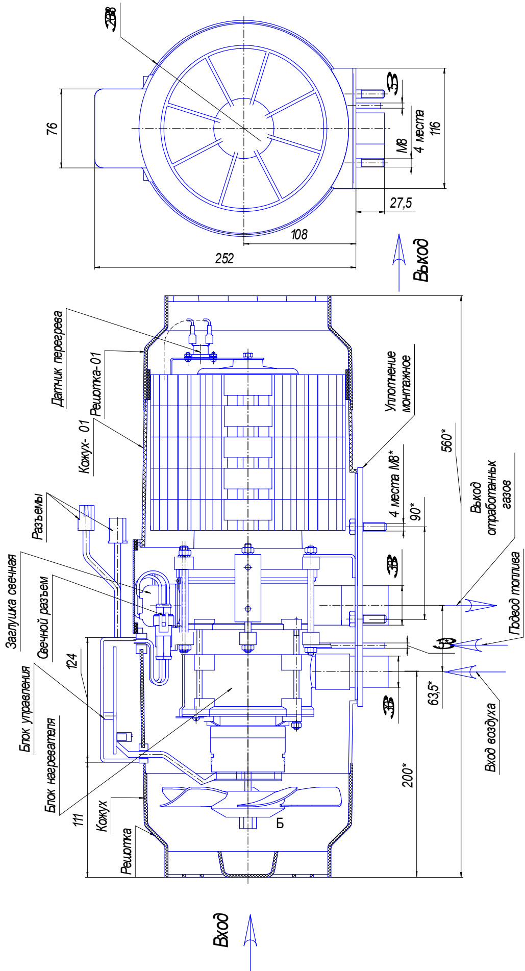
Рисунок 3 – Основные узлы нагревателя
