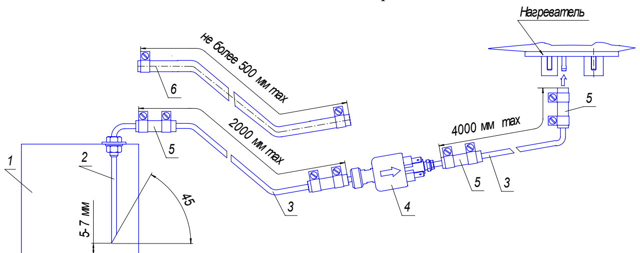
Рис. 8 – Монтаж топливозаборника.
